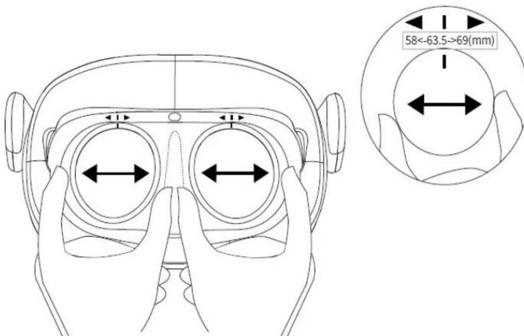
Рисунок 41 — Регулировка расстояния между зрчками
